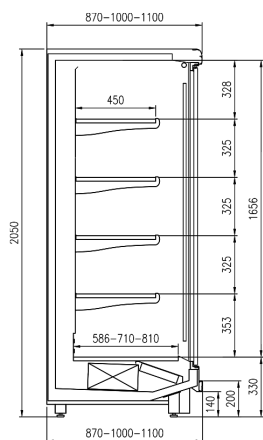
VENEZIA H205 Ecovision
